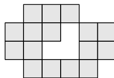
Figure 1: A polyomino.
